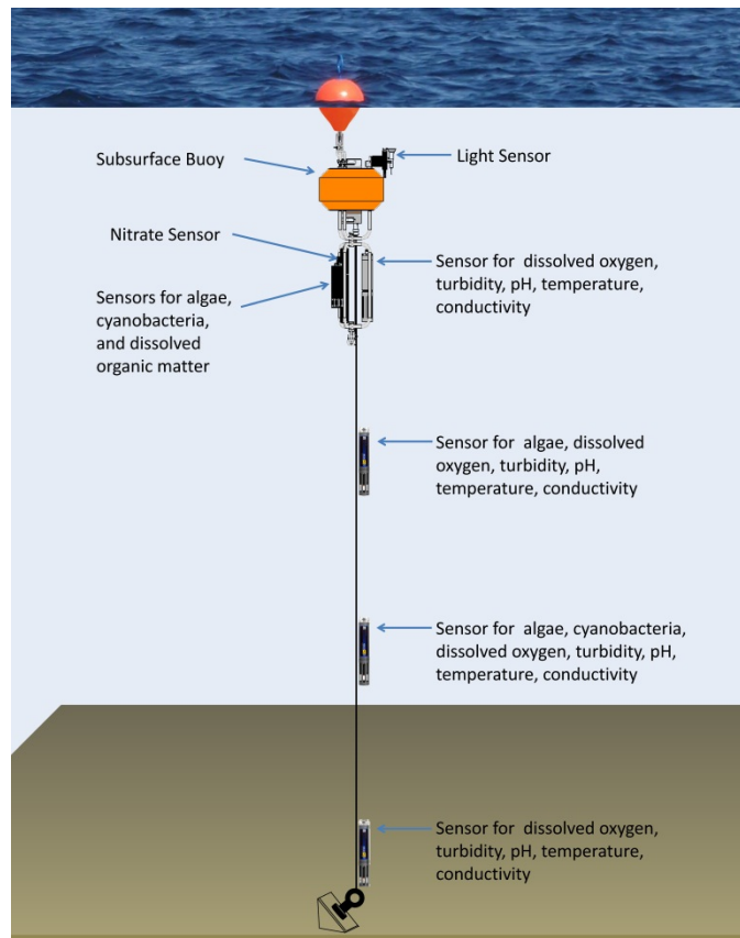
Sensor string
